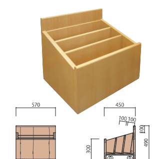
紙芝居架 キャスター付
