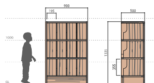
紙芝居架 A型
