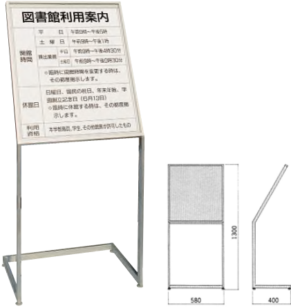
図書館利用案内板 4900 W580 × D400 × H1300 ¥223,000+税 画面サイズ: W550×H700 表示基板: アクリル 表示基颜色: アイボリー フレーム: ステンレス 解説方式: ケンドン ※印刷変更可能です。
