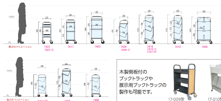
パンチングブックトラック 傾斜片面3段 特注可能 7429 片面 W700×D340×H1175 棚間隔 上段340、下段340、棚奥行250 キャスター100φ、耐荷重150kg程度 ※価格は別途ご相談ください。
