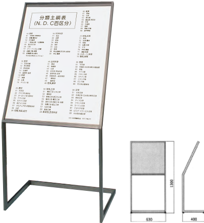
NDC主綱表第9版 スタンド型 4292 W630 × D400 × H1300 ¥242,000+税 画面サイズ: W600×H775 表示基板: アクリル 表示基颜色: 白 フレーム: スチール焼付 ※NDC第10版の対応も可能です。
