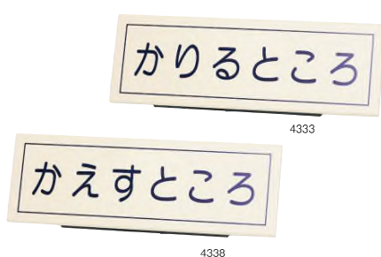
受付案内板児童用 4333 かりるところ W240×D60×H80 ¥15,400+税 4338 かえすところ 画面サイズ: W240×H80 表示基板: アクリル 着脱方式: スライド 表示基板色: アイボリー、ダークグレー フレーム: スチール (t=1.2) 焼付塗装
