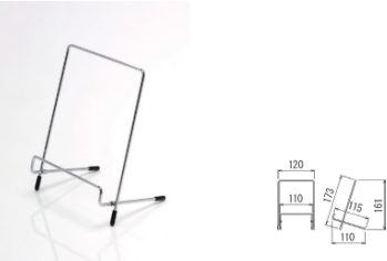
展示スタンド 200 4183 W120×D110×H161 ¥1,000+税 A5-B5サイズ対応
