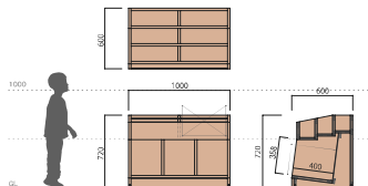
紙芝居架 B型
